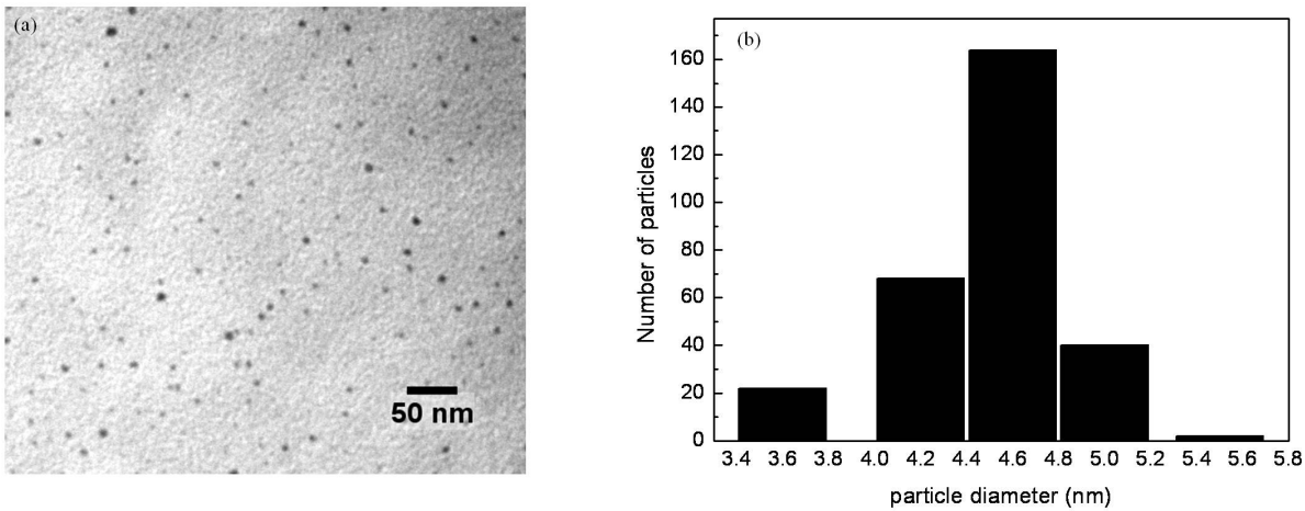
Figure 8.9: Image TEM (a) et la distribution correspondante (b) des nanoparticules de Au-PNIPAM 265 synthétisées par la méthode du "one-step" en utilisant le rapport HAuCl_4:Polymère = 10:1 .
