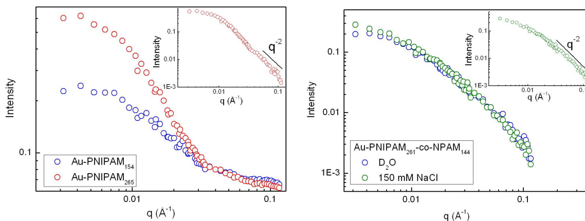
Figure 8.10: Courbes de diffusion des nanoparticules de (a) Au-PNIPAM 154 (bleu) et Au-PNIPAM 265 (rouge) dispersées dans le D 2 O et (b) Au-PNIPAM 261 -co-NPAM 144 dispersées dans le D 2 O en absence (bleu) et présence de NaCl (vert) (T = 20°C. Insets: pente en q^{-2} pour les courbes de diffusion après soustraction du bruit de fond).
