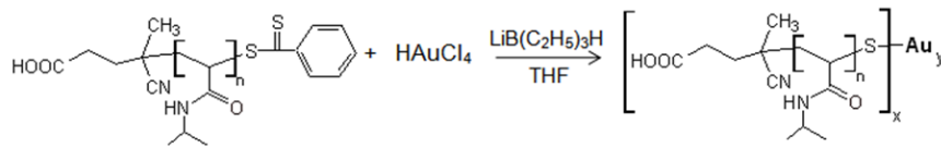
Figure 8.8: Synthèse des nanoparticules d'or Au-PNIPAM.
